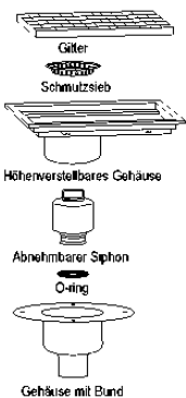
Dezentraler Abfluss mit höhenverstellbarem Gehäuse
