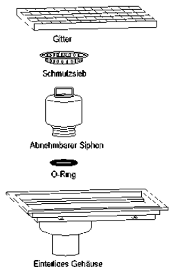
Dezentraler Abfluss mit einteiligem Gehäuse
